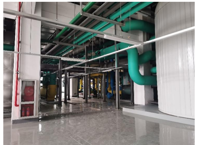
制冷机房
